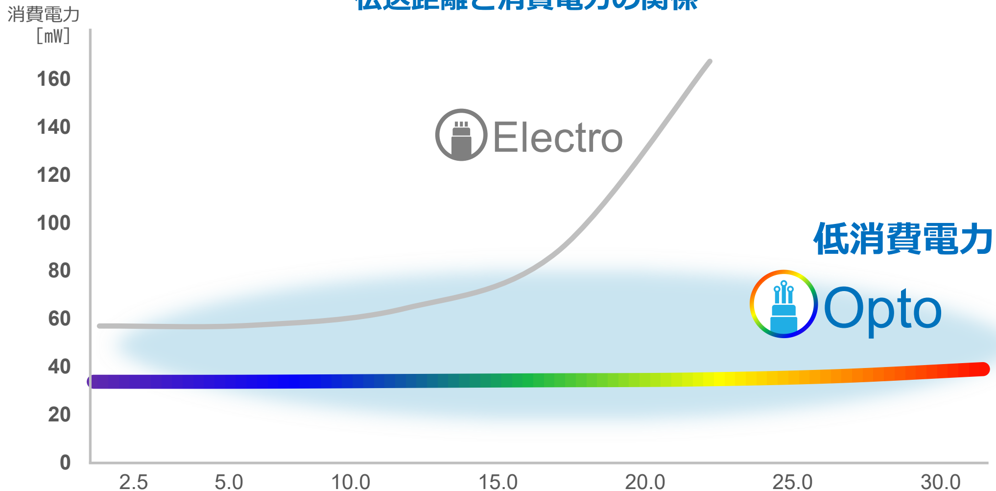
伝送距離と消費電力の関係
