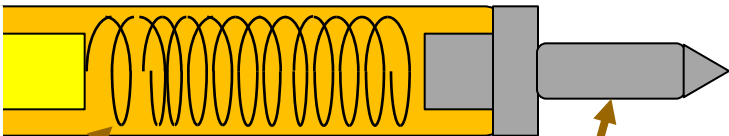
コンタクトプローブの簡略図
