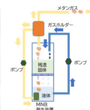
TOSS®ハイブリッドメタン発酵システム図
