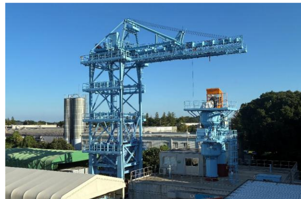
「テックファーム」における 排土設備（ABキャリア）
